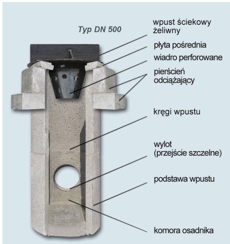
Rys. nr 2 – Kompletny studzienka ściekowa wraz z wpustem ulicznym.
