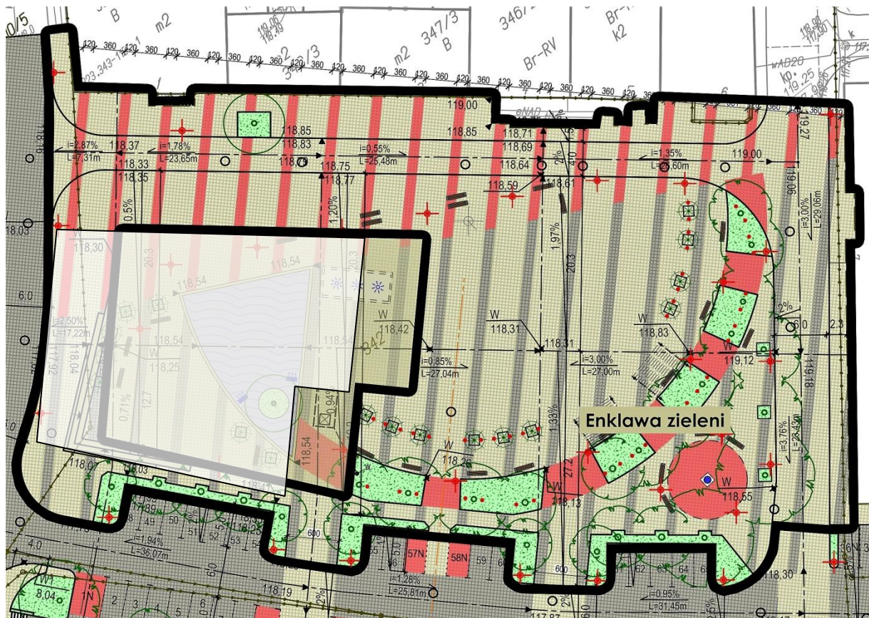
Wyrys z dokumentacji (planowany zakres przebudowy)
